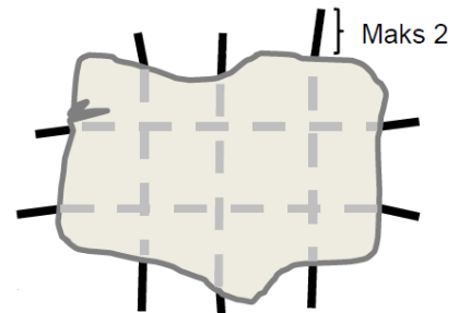
Figur 1 Armeringsjern må maksimalt stikke 2 cm ud over betonen
